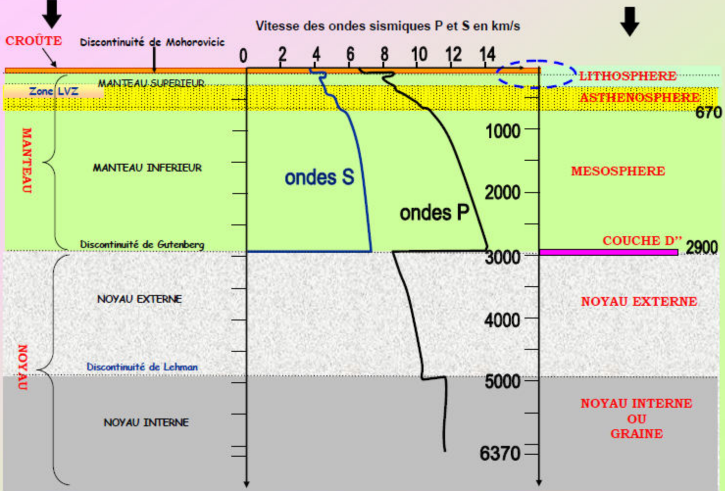
Profondeur de la Terre en km
